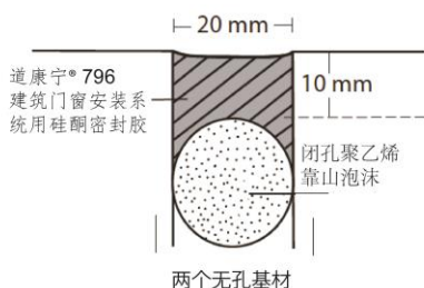
图2：浅接缝
