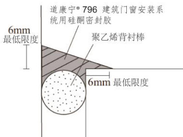
图3：角接缝
